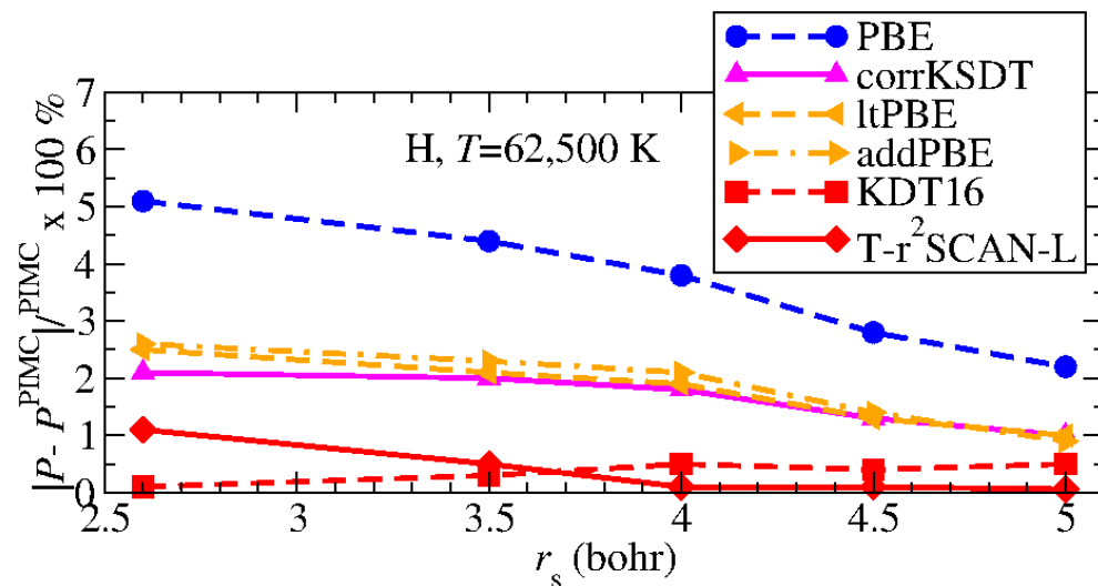
Relative error DFT vs fermionic PIMC
